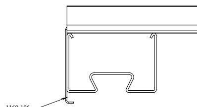
AMRPK otsakandur kõrge klambriga
